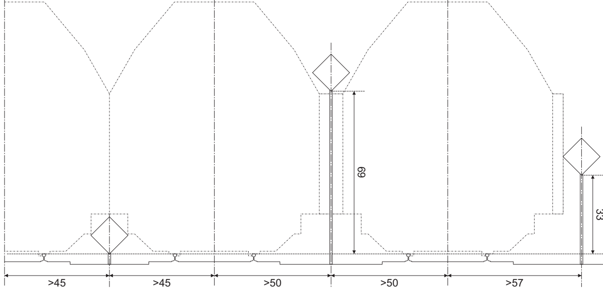
Wskaźniki dla linii zelektryfikowanych EI 1-EI 6, K 8b
