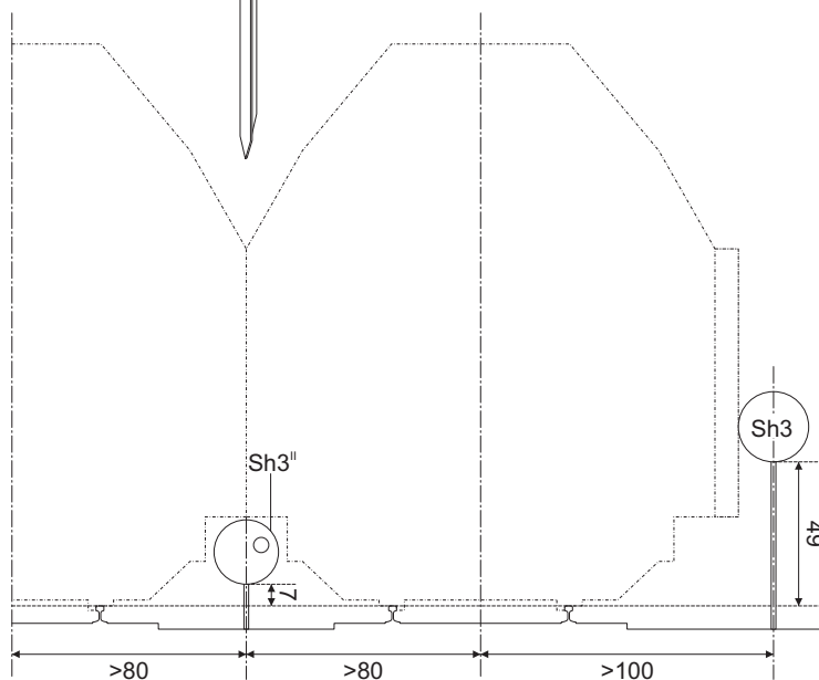
Stelaż do sygnalów Lf 1, Sh 2, Sh 3 (wariant)
