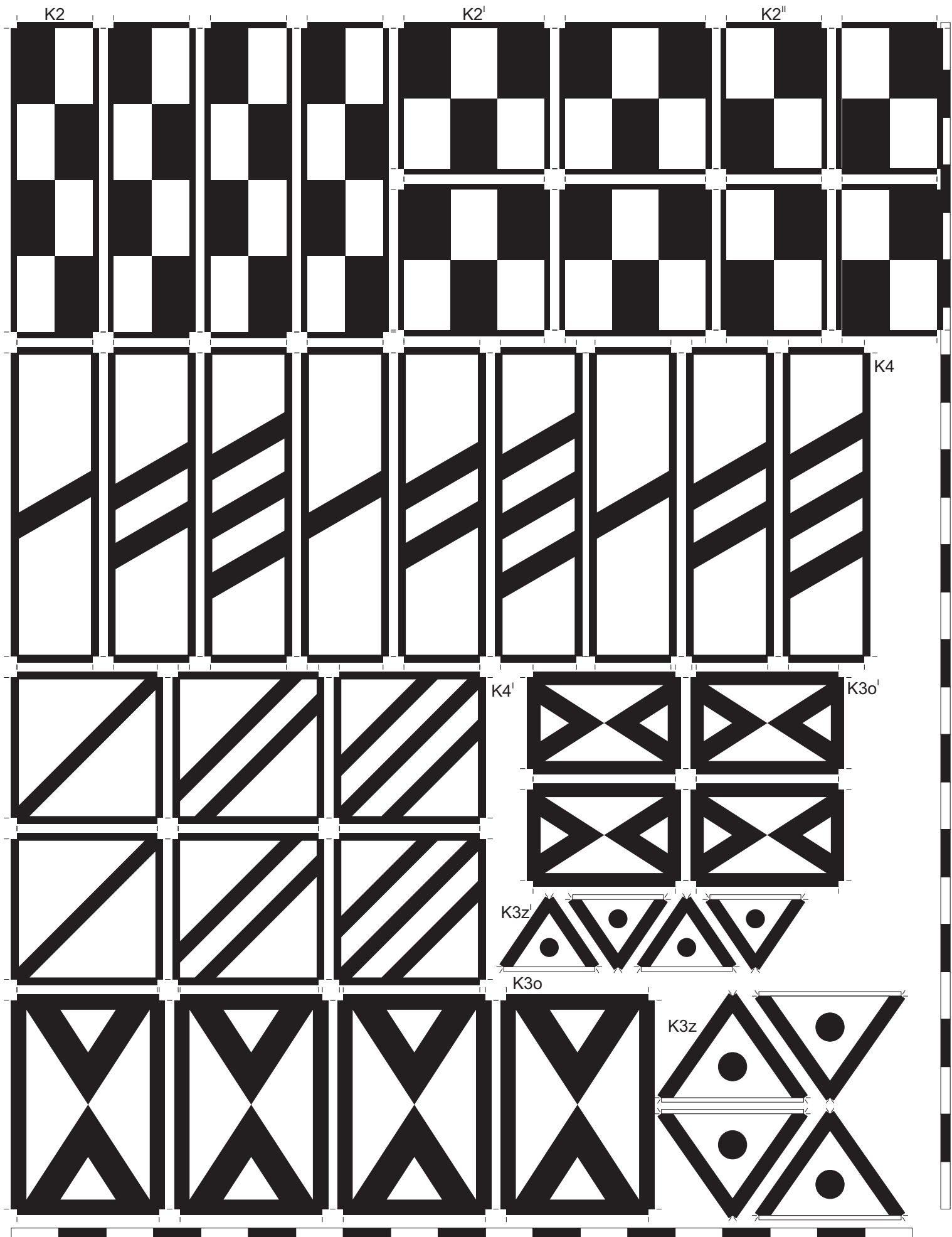
Wskaźniki kolejowe DRG/DR, 1935-1945, skala 1:25
