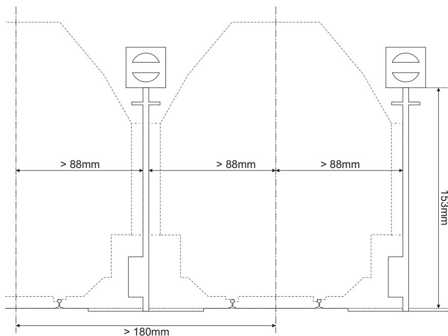
Umieszczenie tarczy względem skrajni
