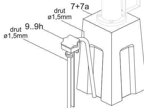
Fundament metalowy
