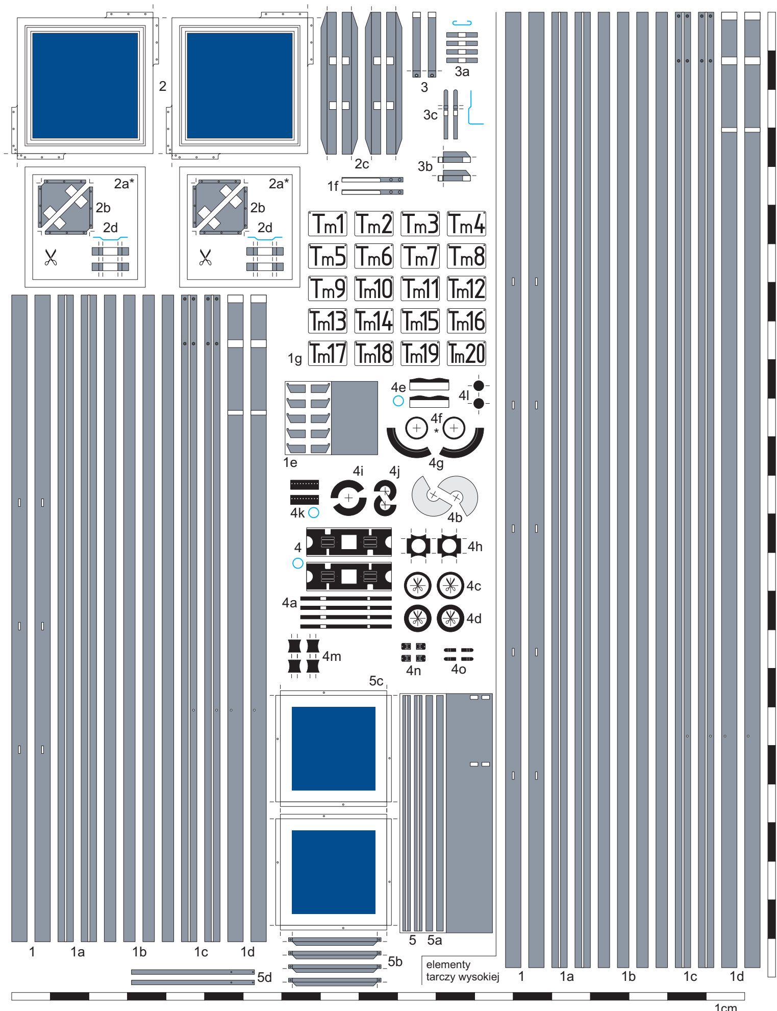
Tarcza manewrowa stała, skala 1:25
