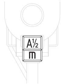
Umieszczenie dodatkowej tabliczki dla sygnału manewrowego
