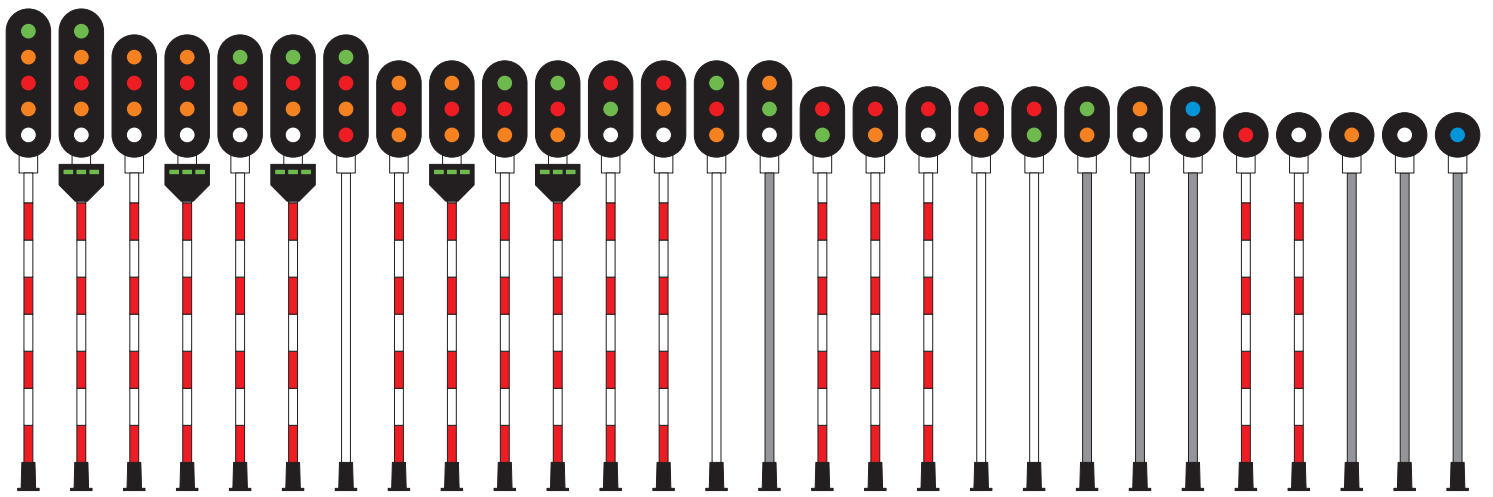
Typowe układy barw komór sygnalizatorów PKP (pas świetlny może być zielony, pomarańczowy lub dwukolorowy).
