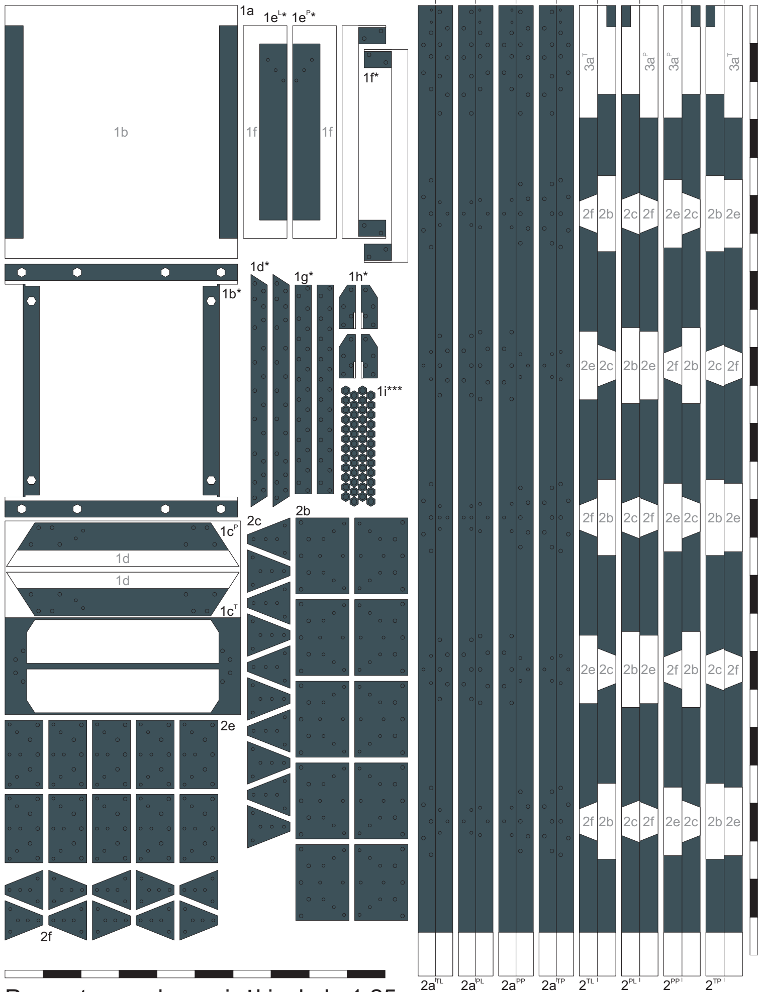
Pomost sygnałowy ciężki, skala 1:25
