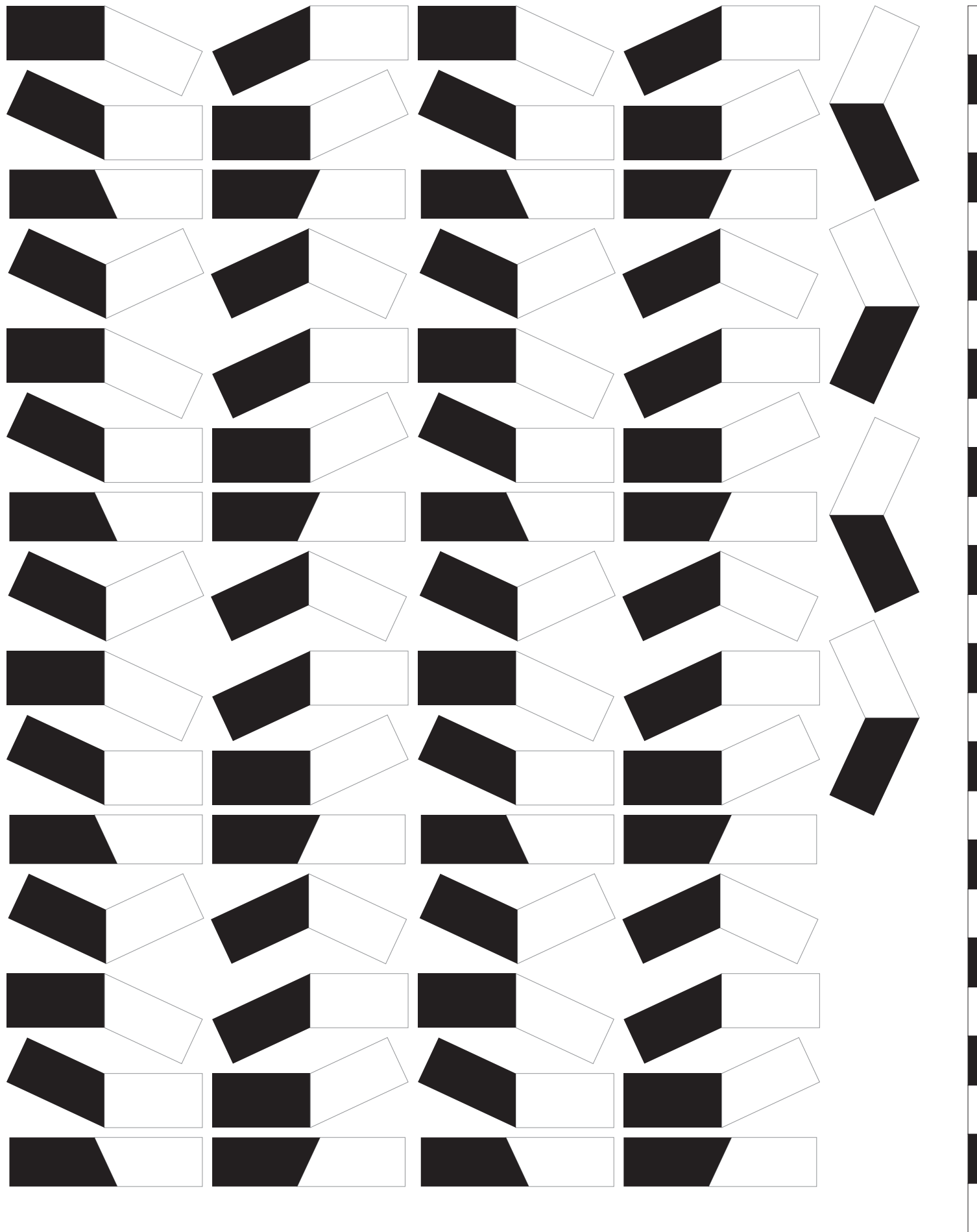
Znaki pochylenia podłużnego PKP, skala 1:25 1cm
